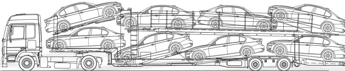
Beladebeispiel ruslan® mit 4,00 m Höhe. Nationale Vorschriften sind zu beachten!
