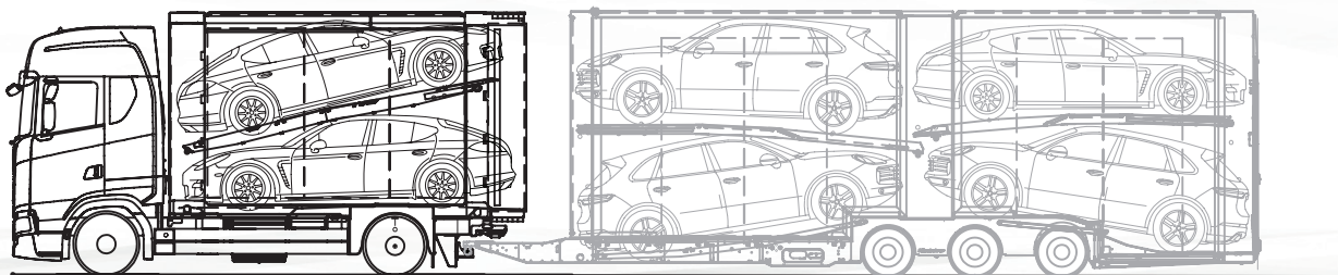
Beladebeispiel ecomode performance S2-180 in Kombination mit ecomode performance T4-235 mit 4 m Höhe. Nationale Vorschriften sind zu beachten!
