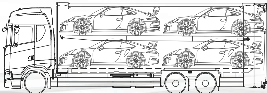
Beladebeispiel ecomode performance S4-260 L mit 4,00 m Höhe. Nationale Vorschriften sind zu beachten!
