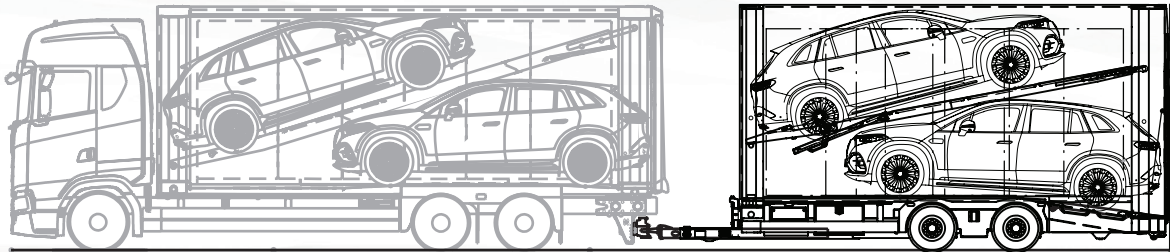
Beladebeispiel ecomode performance S2-260 in Kombination mit ecomode performance T2-180 mit 4 m Höhe. Nationale Vorschriften sind zu beachten!
