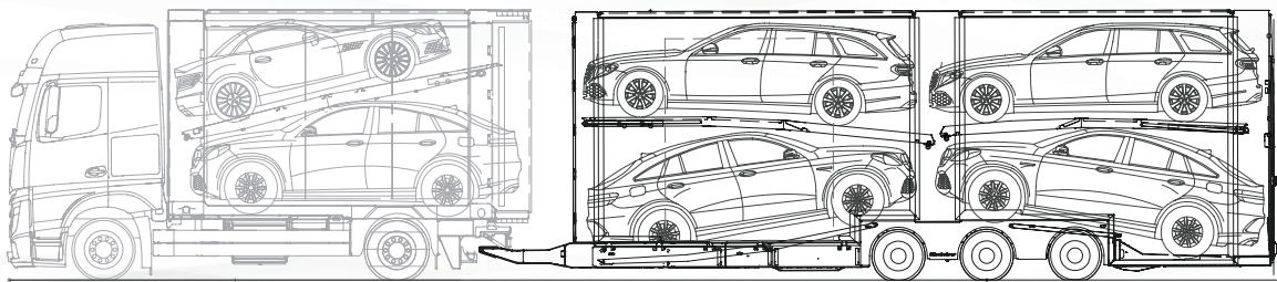
Beladebeispiel ecomode performance S2-180 in Kombination mit ecomode performance T4-235 mit 4 m Höhe. Nationale Vorschriften sind zu beachten!
