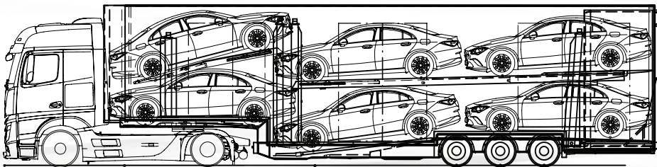
Beladebeispiel ecotrans performance 6-250 mit geteilter Hebebühne mit 4 m Höhe. Nationale Vorschriften sind zu beachten!
