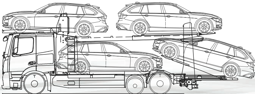
Beladebeispiel variotrans® pro Typ A4 mit 4,00 m Höhe. Nationale Vorschriften sind zu beachten!
