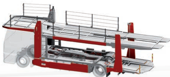
variotrans® pro A4
