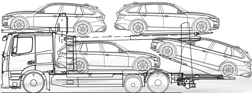
Ejemplo de cargavariotrans® pro tipo A4 con 4,00 m de altura. ¡Respetar las prescripciones nacionales!
